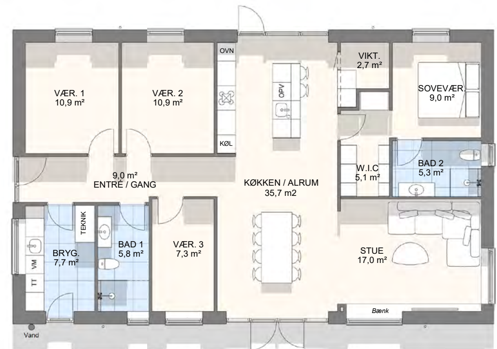
K2 VALUE CONCEPT PLANTEGNING 150 M 2 FRA KR.2.100.000
